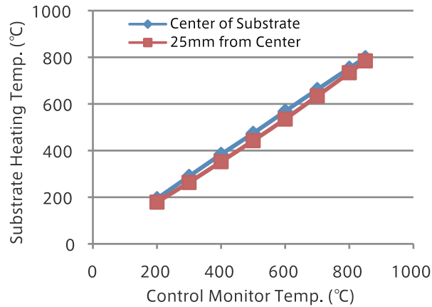
基板加熱特性
