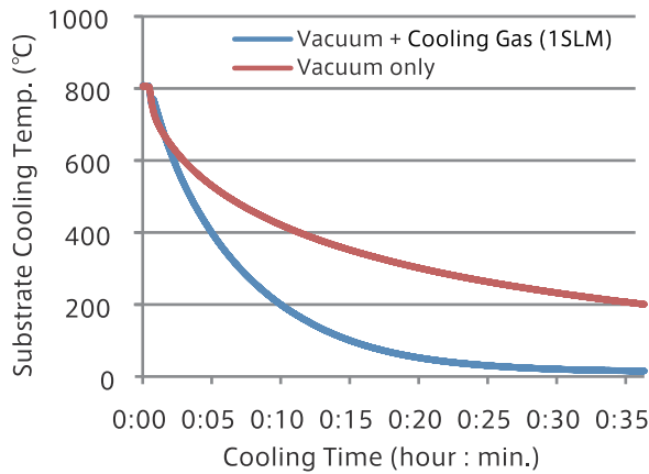
基板冷却特性
