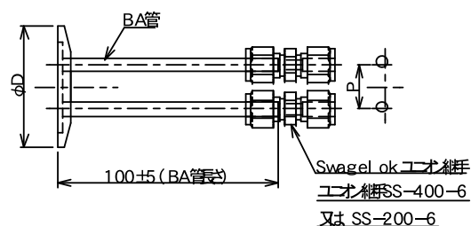
●NWフランジ-φ1/8パイプアダプタ
